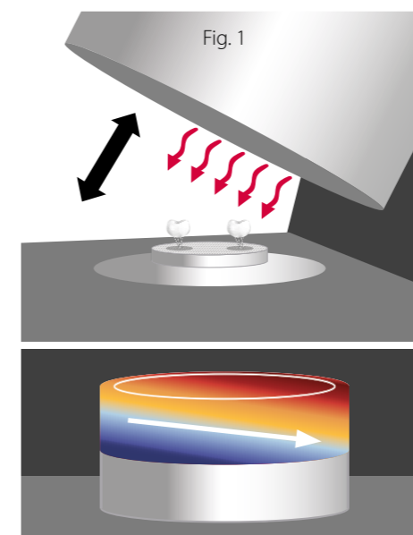
Fechamento angulado: Distribuição irregular de calor na bandeja e nos elementos posicionados.
